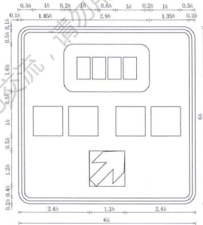
图 D. 64 [图 261d)]
