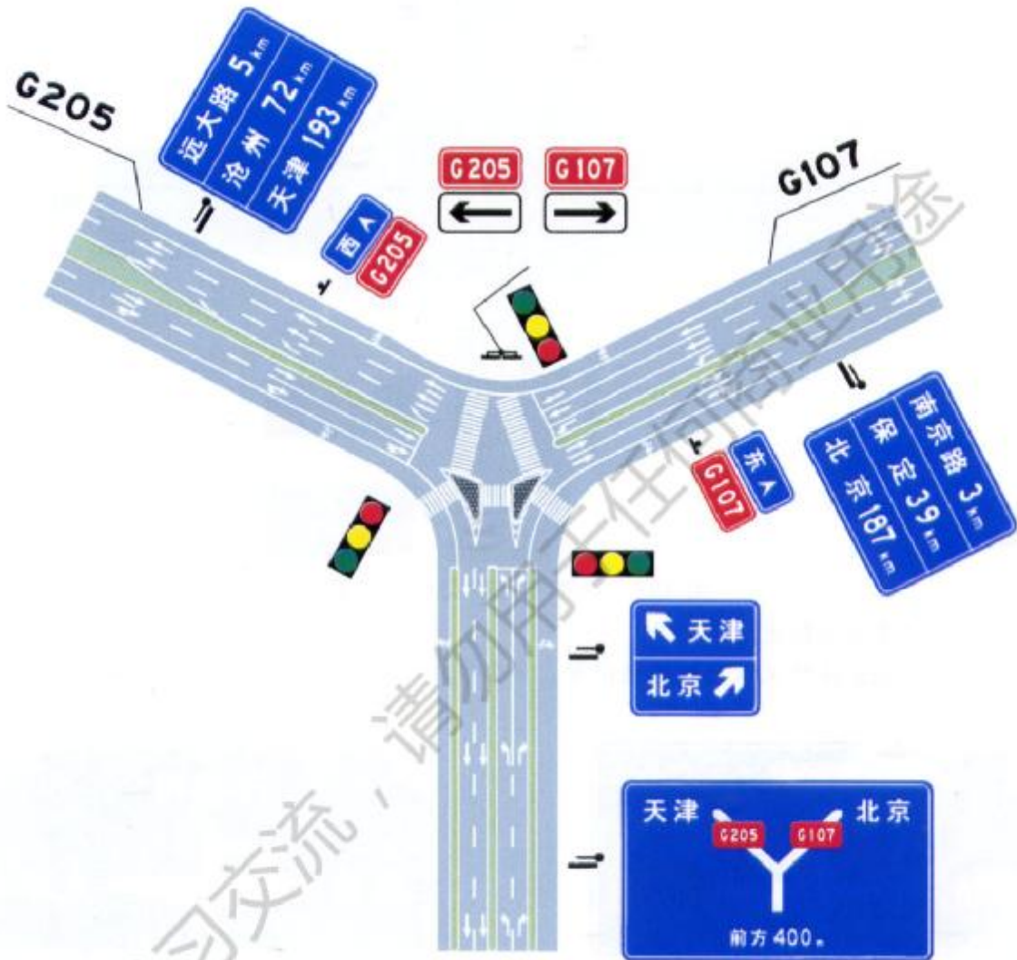
图 195 Y 型交叉路口标志设置例
