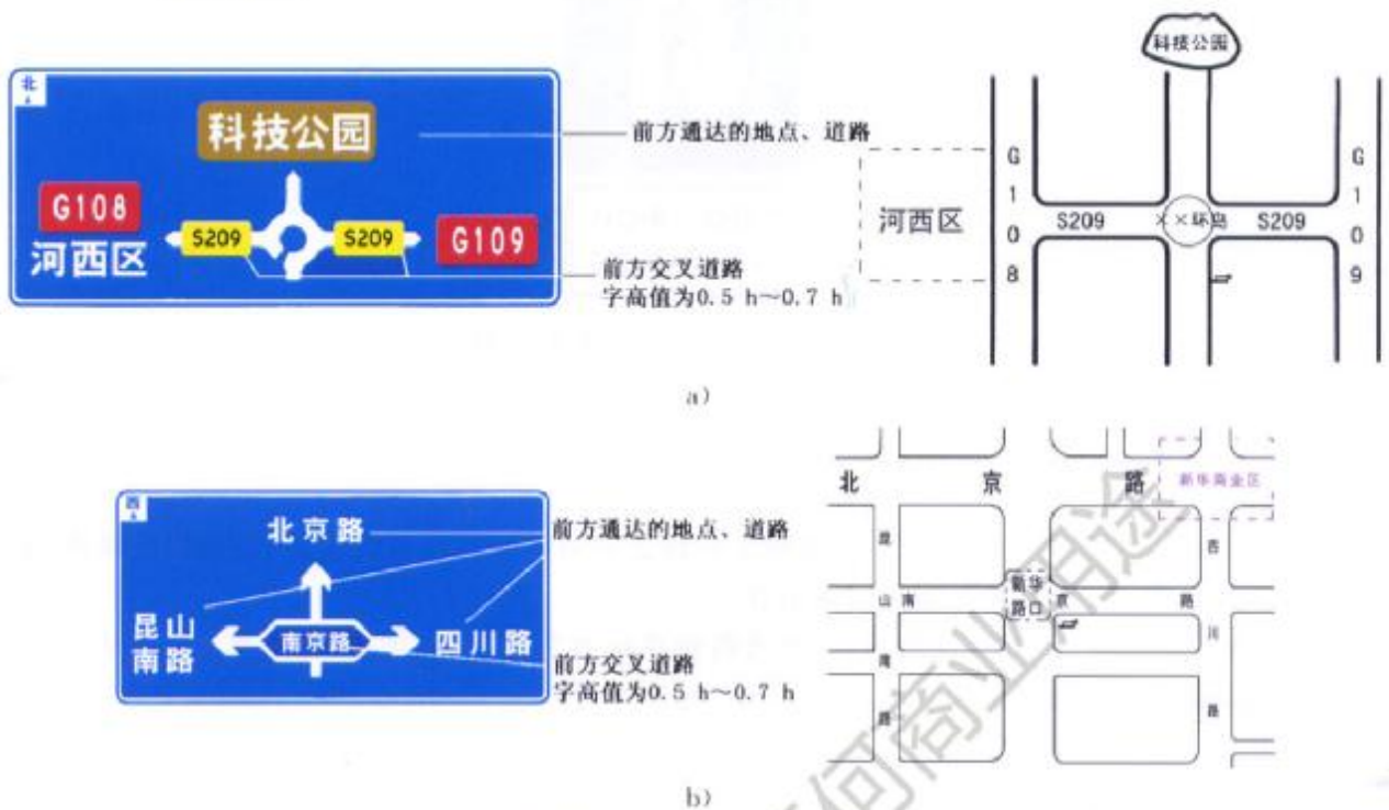
图 184 标志信息示例
