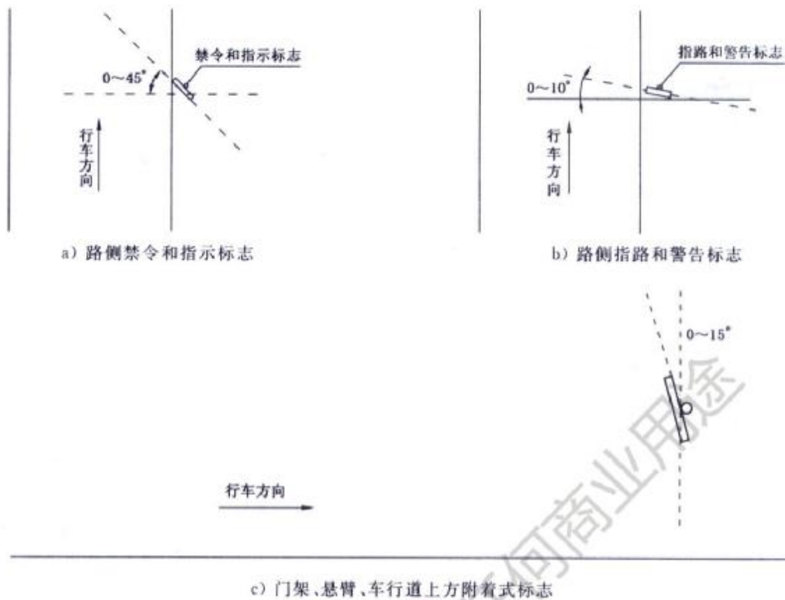
图 6 标志安装角度示意
