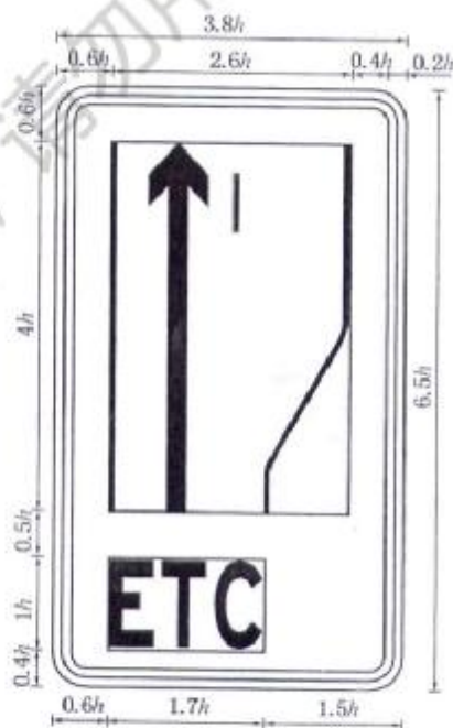
图 D. 103 [图 285b)]
