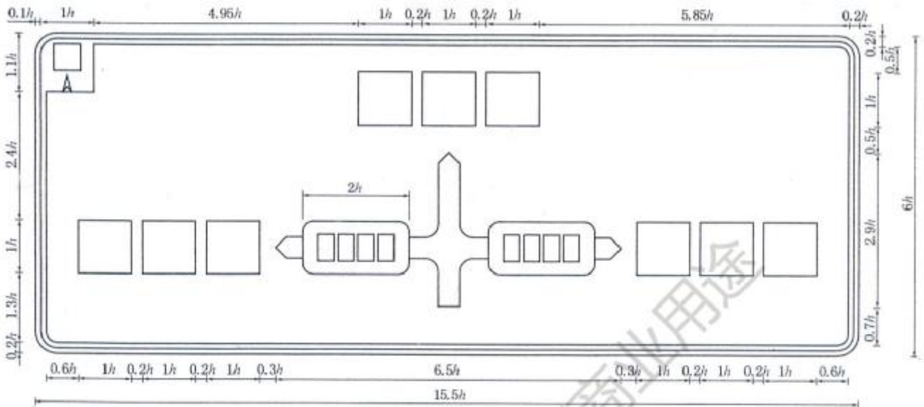
图 D.11 [图 192b)]
