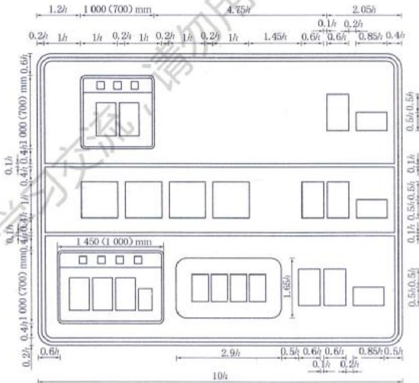
图 D.54 [图 258b)]
