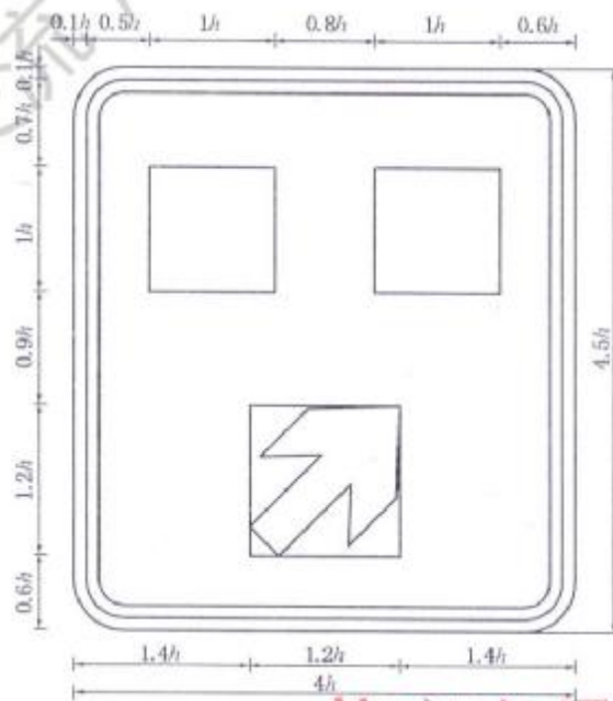
图 D.68 [图 263a)]
