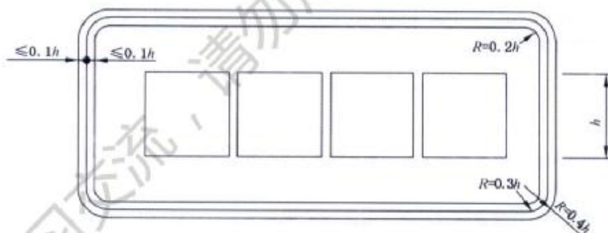
图5 外边框和衬边尺寸
