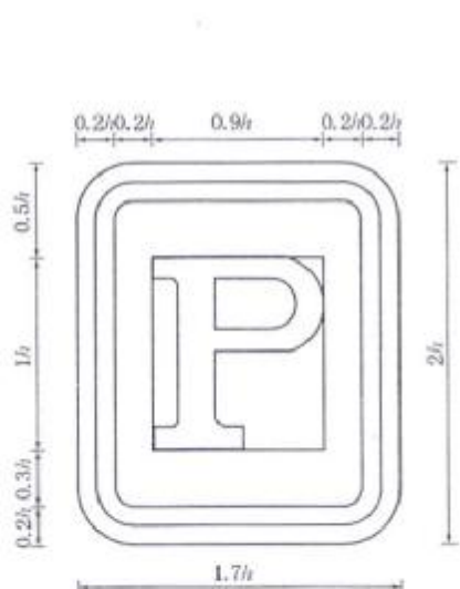
图 D. 114 [图 293a)]
