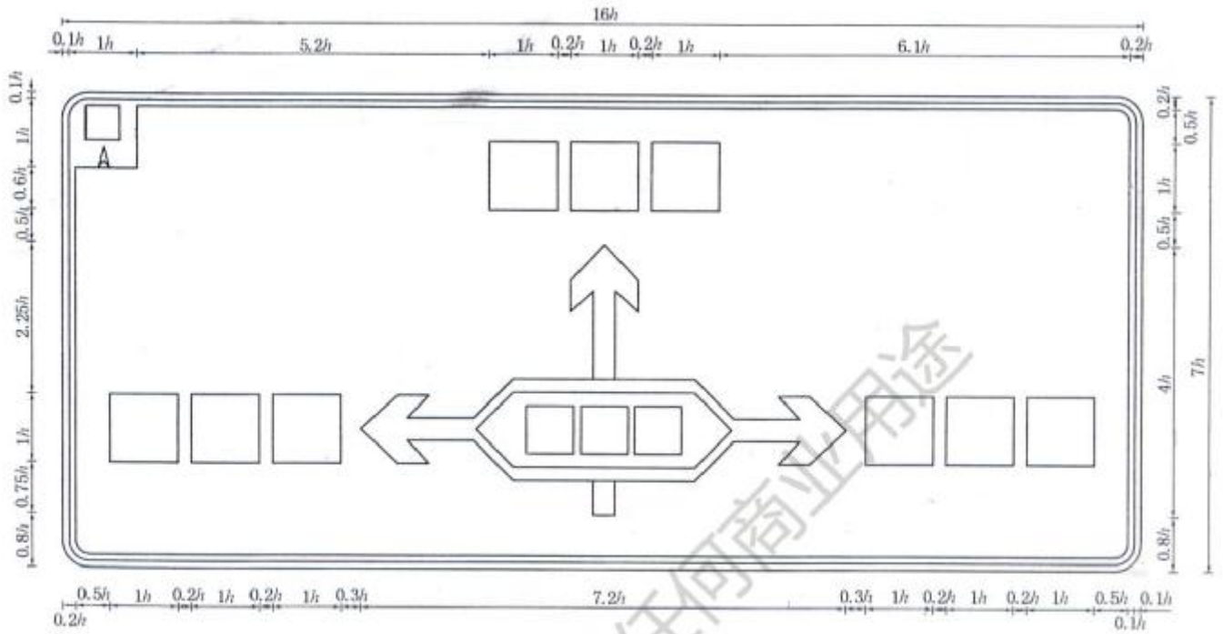
图 D.13 [图 192d)]
