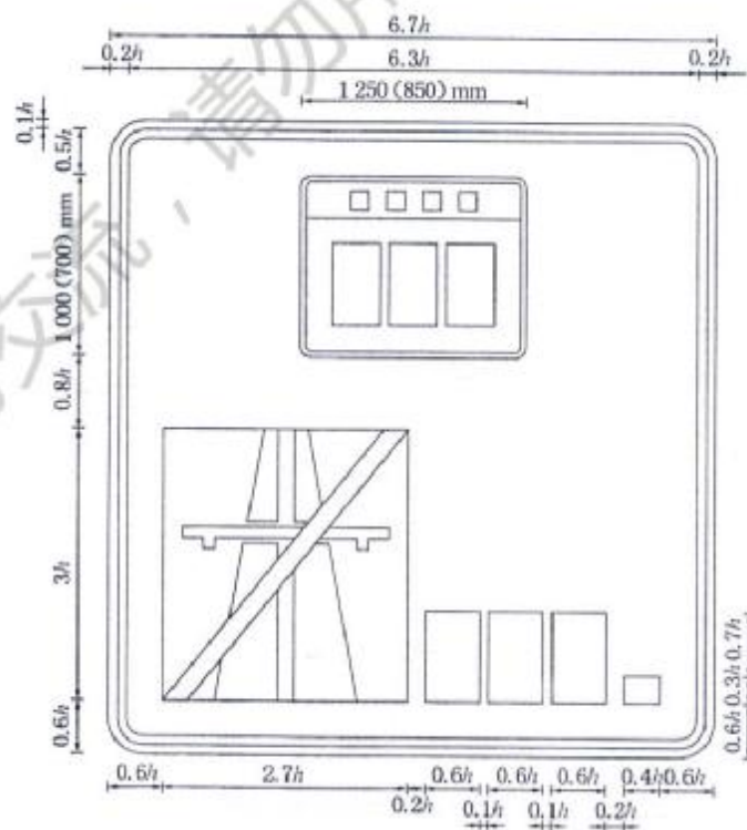
图 D.78 [图 266c)]
