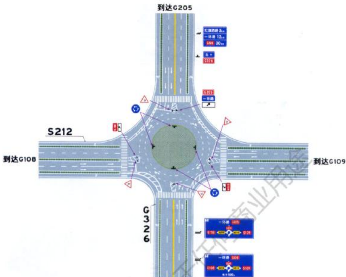
图 197 环形交叉路口标志设置例
