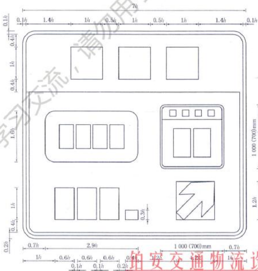
图 D.66 [图 261g)]
