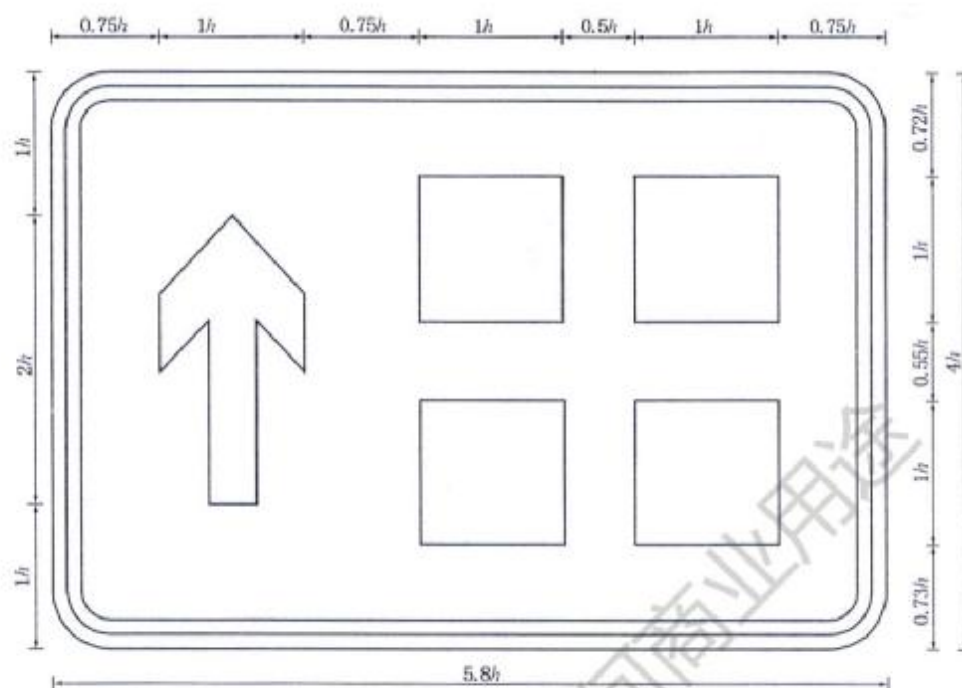
图 D. 69 [图 263b)左]
