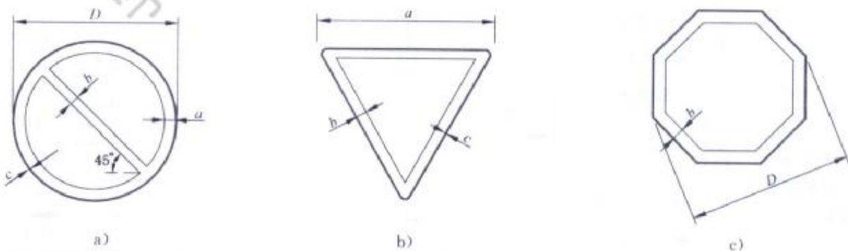
图 3 禁令标志各部分尺寸代号
