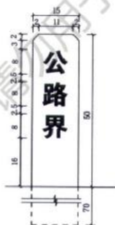
图 248 公路界碑
