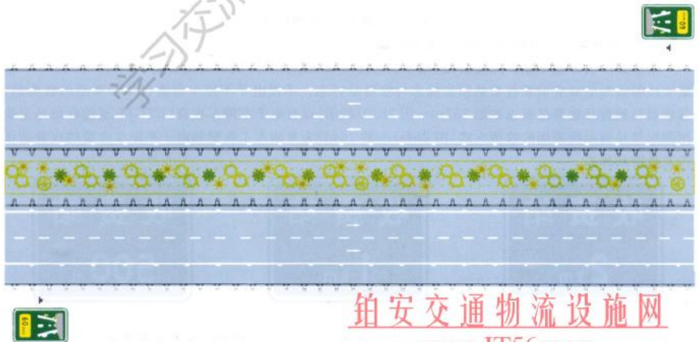
图 279 特殊天气建议速度标志设置示例
