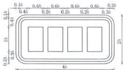
图 D.25 (图 201~图 204)( h 为字母和数字高度)
