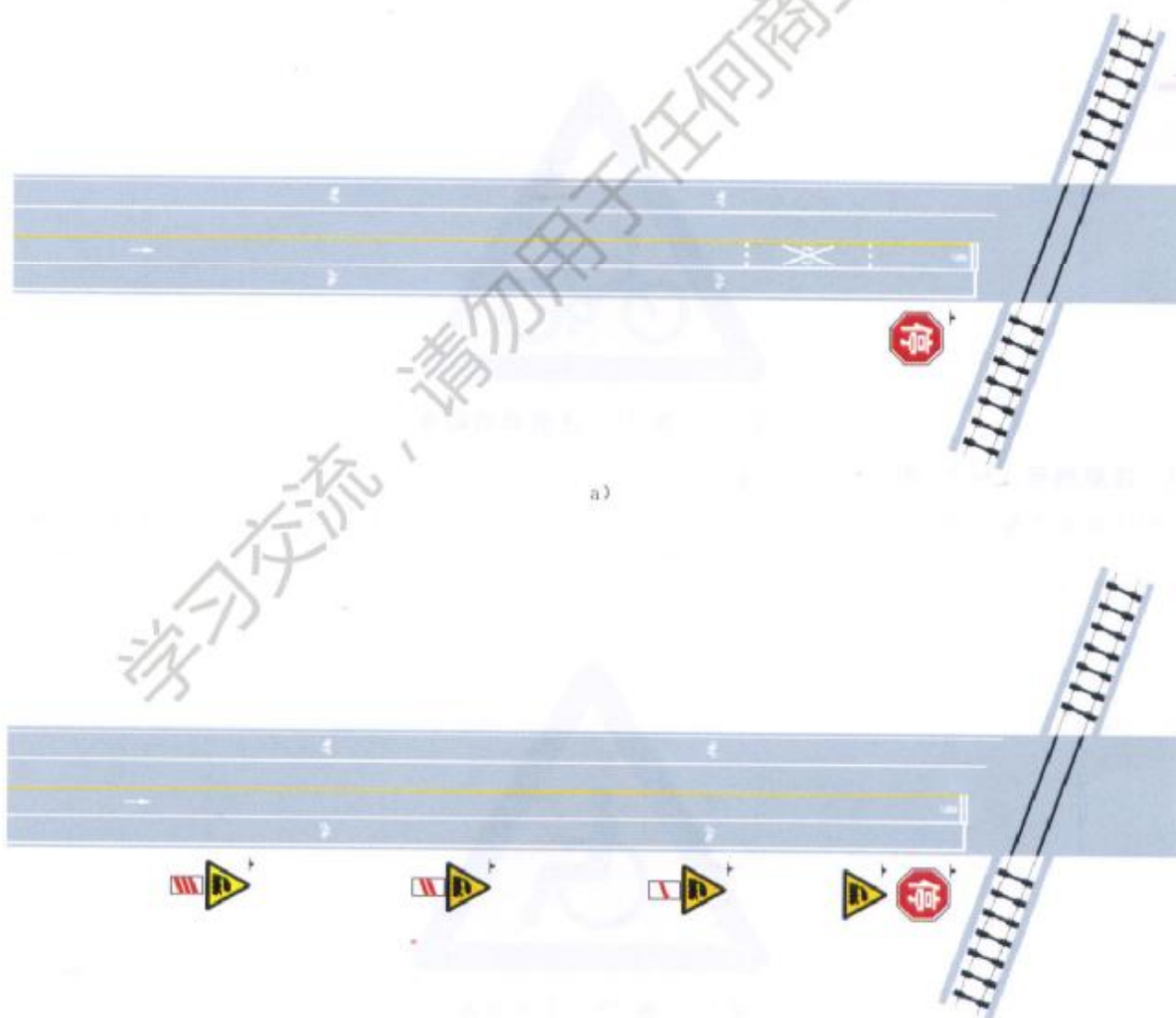
图 50 无人看守铁路道口标志设置示例
