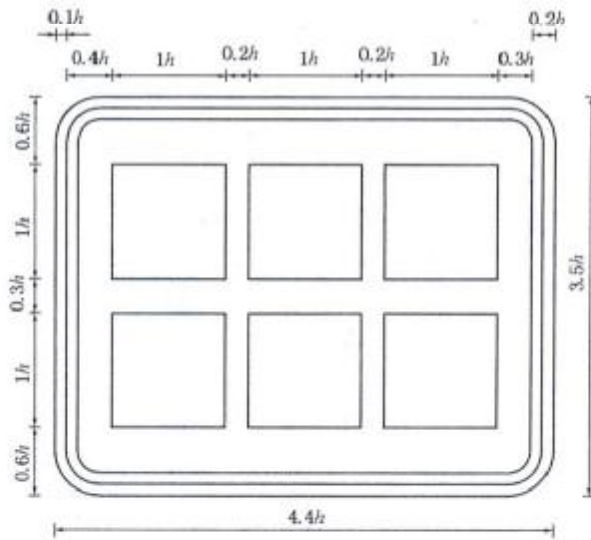
图 D. 26 [图 206a)]
