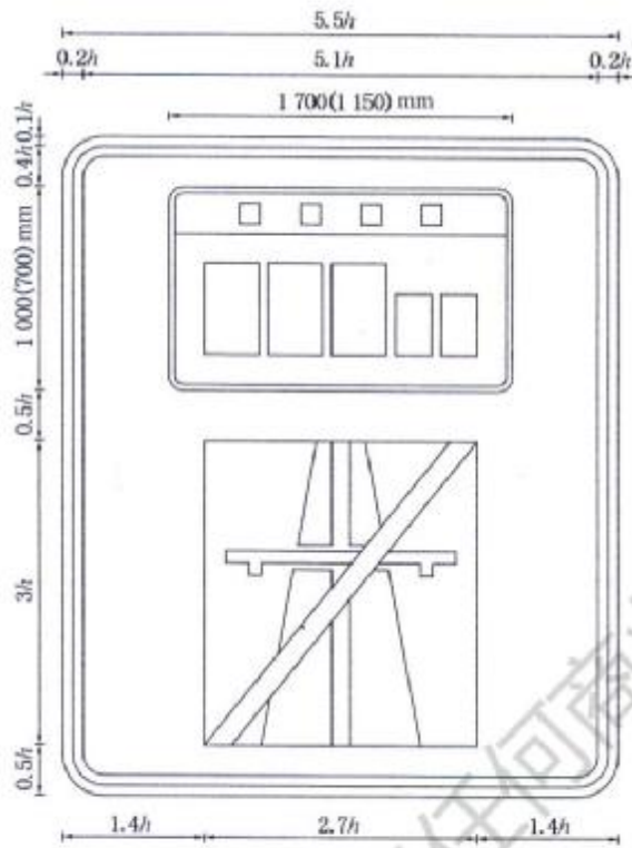
图 D. 83 [图 269b)]
