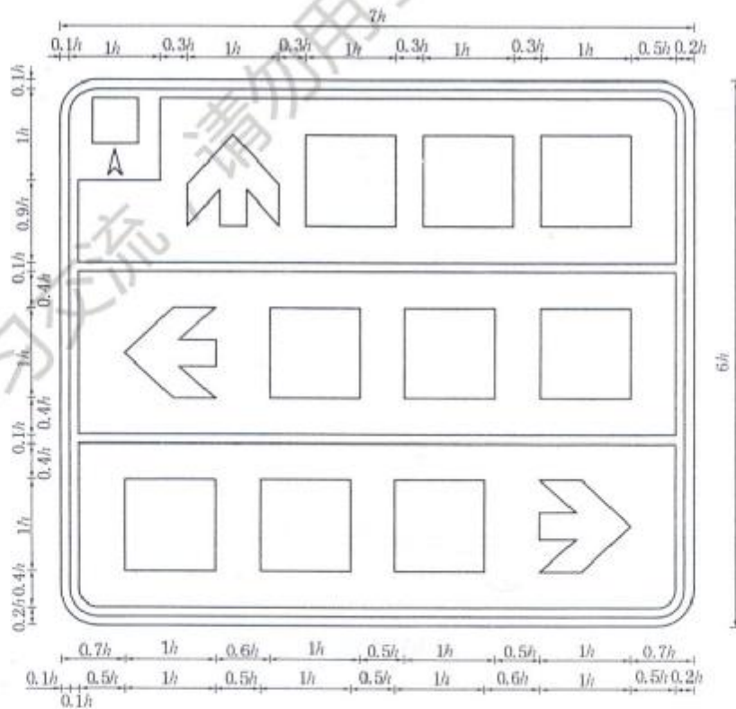
图 D.12 [图 192c)]
