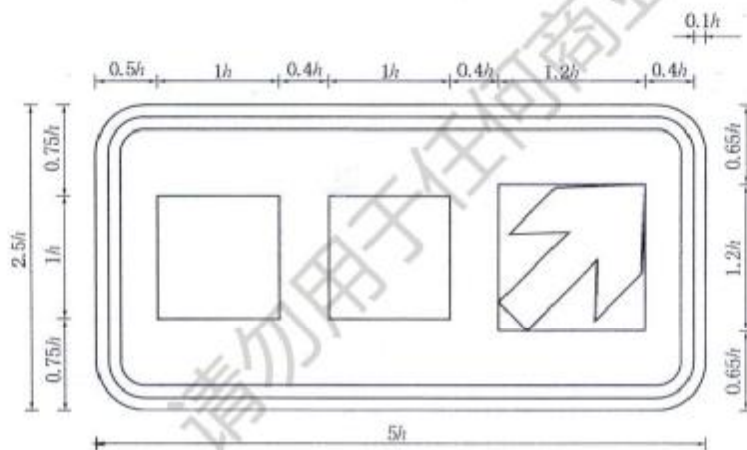
图 D.24 [图 199b)]
