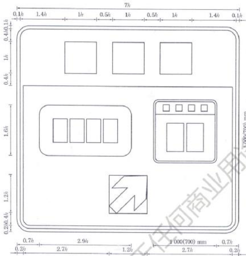
图 D.67 [图 261h]
