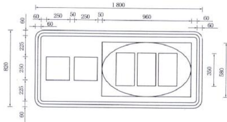
图 D.60 [图 260a)]
