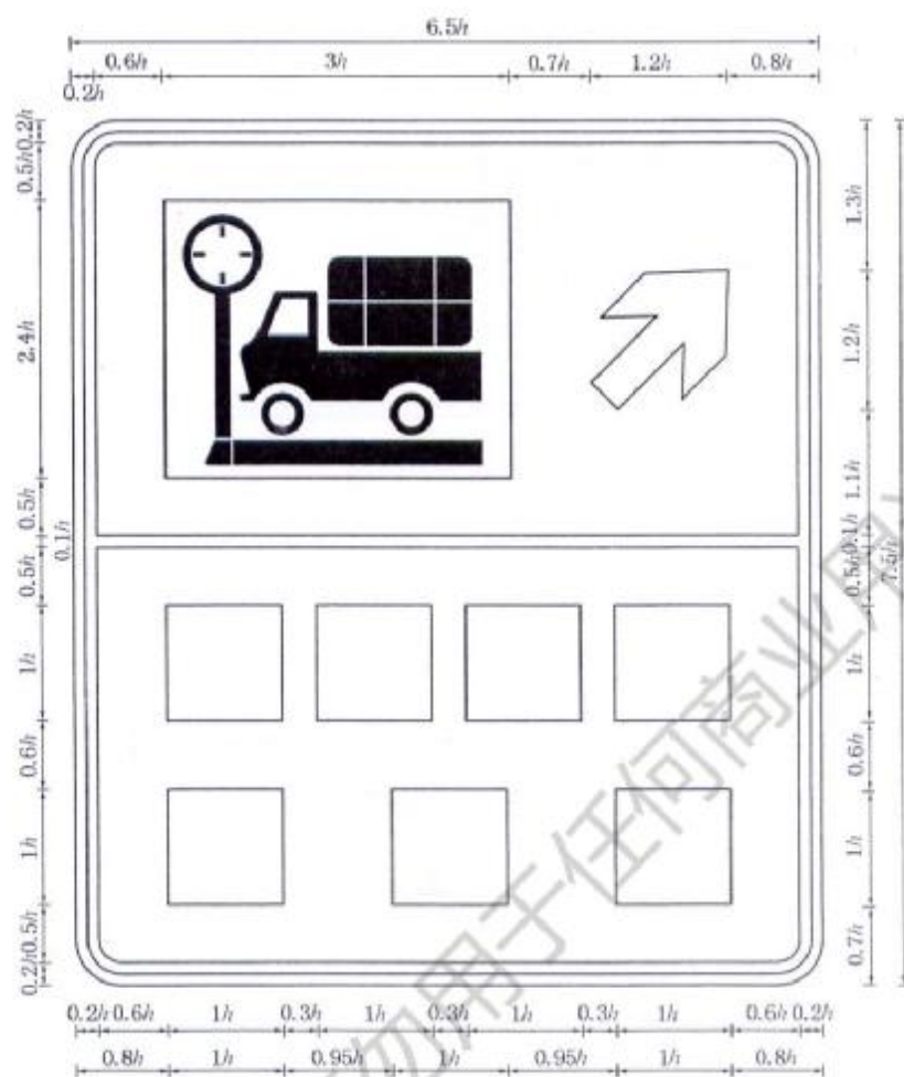
图 D. 122 [图 296d)]
