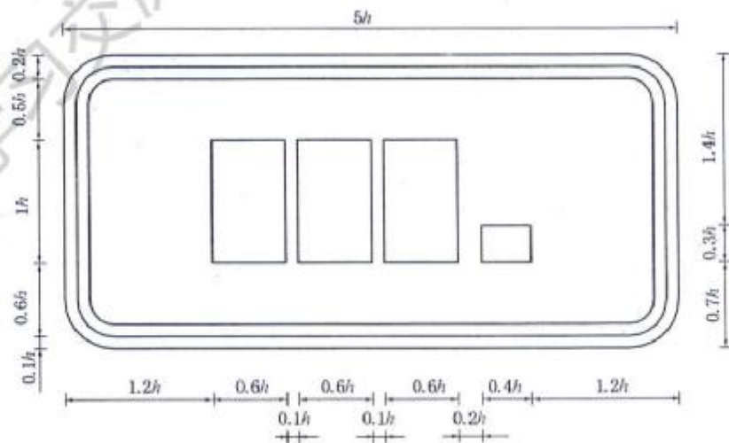
图 D. 93 [图 276e]
