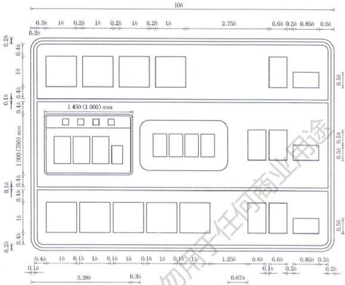
图 D.55 [图 258c]
