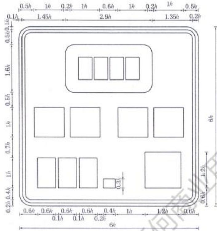
图 D. 63 [图 261c)]
