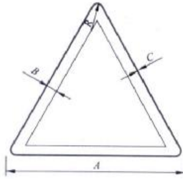
图 2 警告标志尺寸代号
