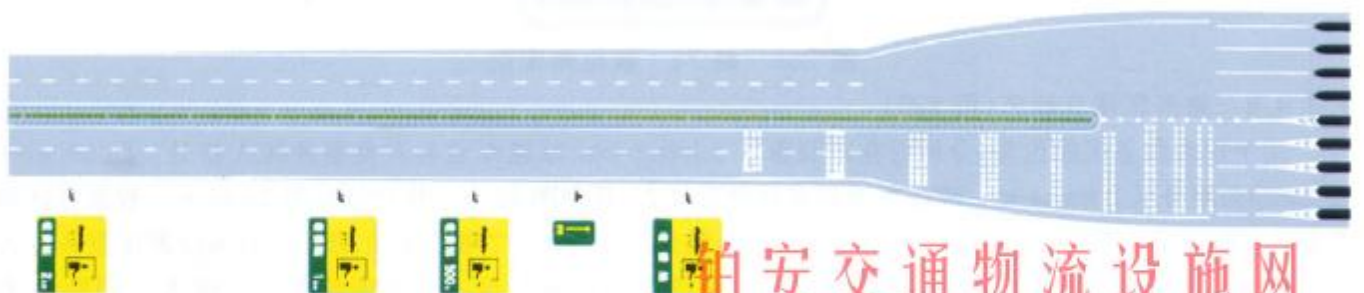
图 286 ETC 车道指示标志设置示例
