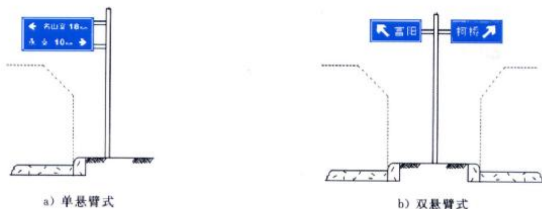
图 8 悬臂式
