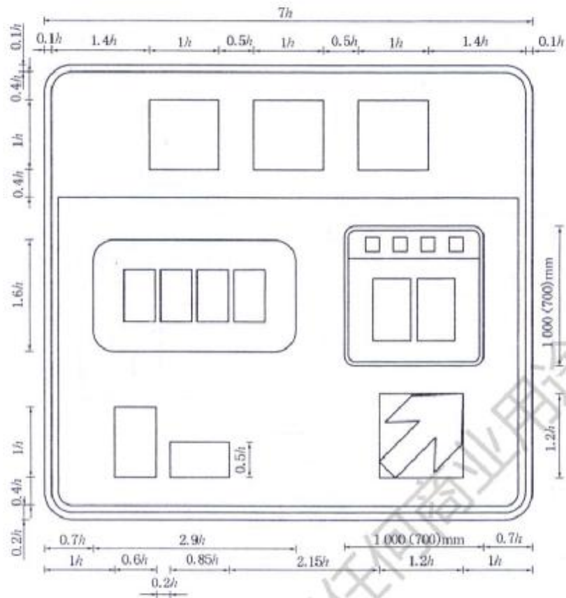
图 D.65 [图 261e)、f)]
