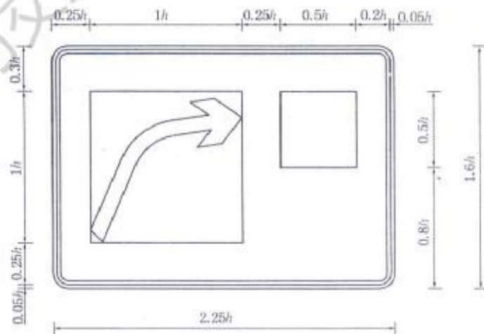
图 D. 123 [图 297b)]
