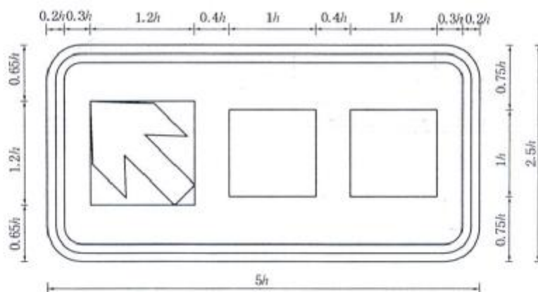
图 D.23 [图 199a)]
