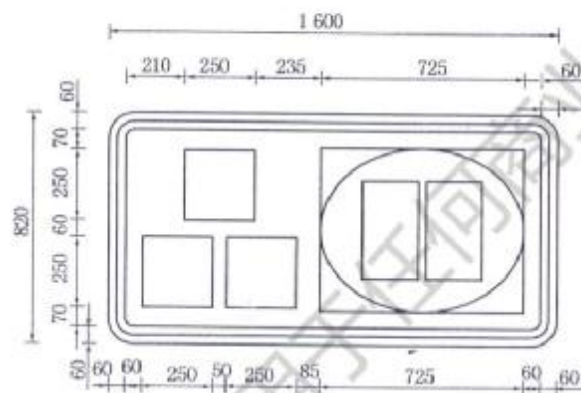
图 D.61 [图 260b)]
