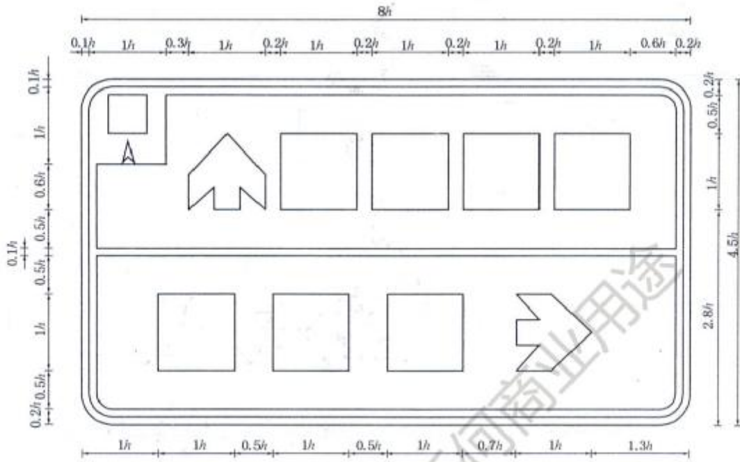
图 D.15 [图 193b]
