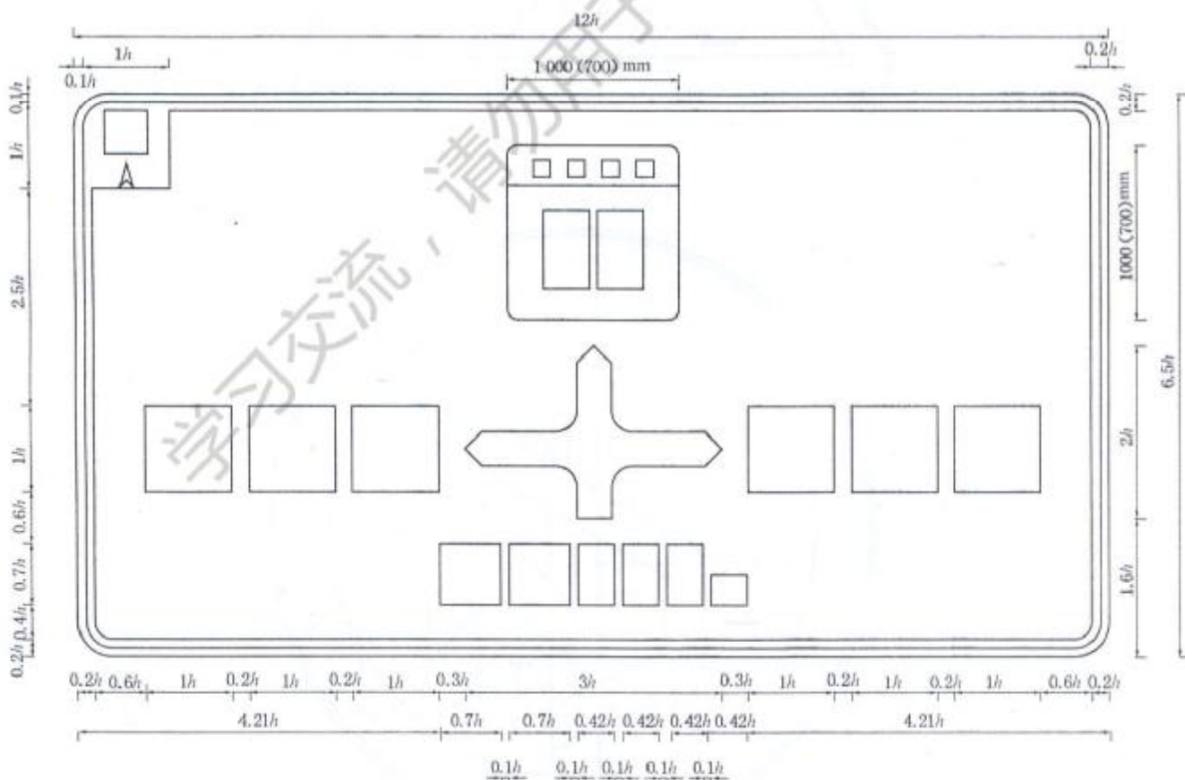
图 D.4 [图 138a]
