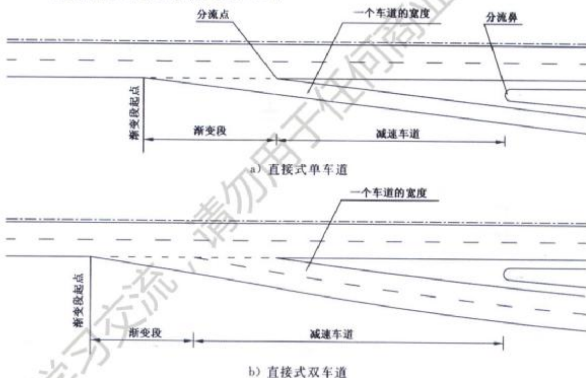
图 187 不同形式减速车道渐变段起点
