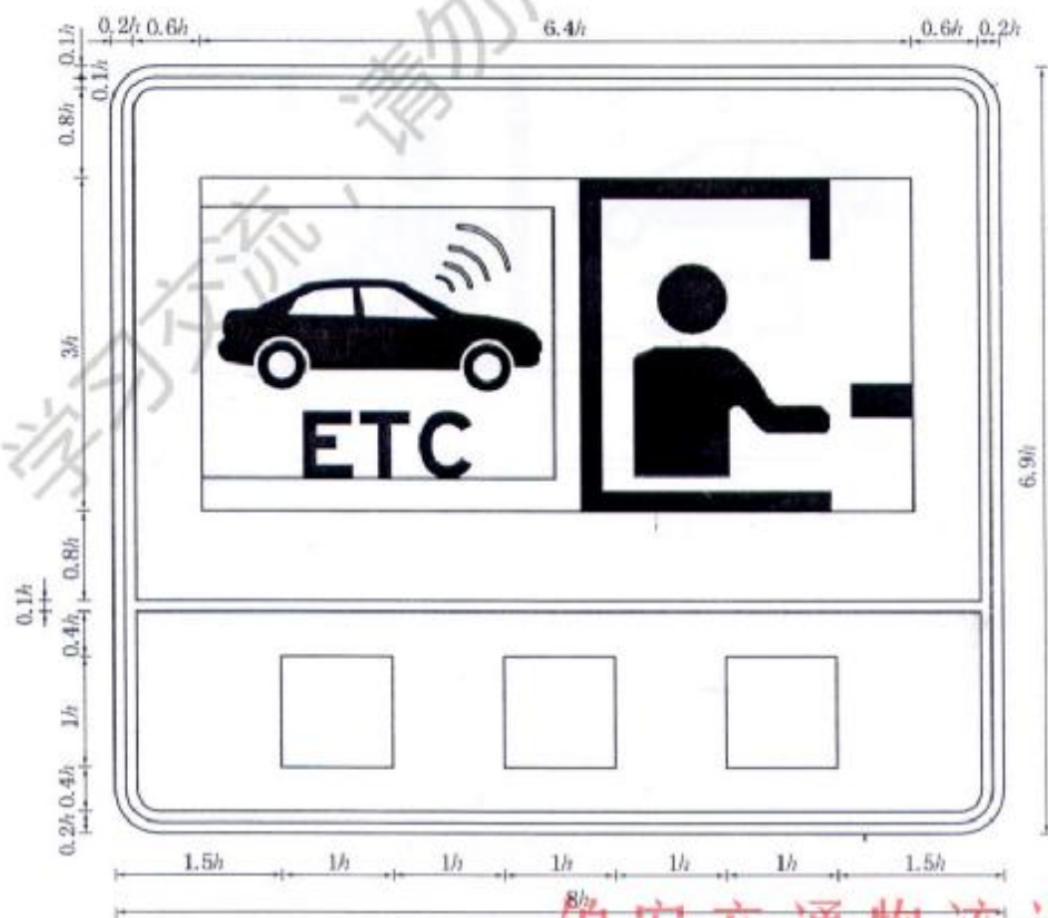
图 D.101 [图 284d)]
