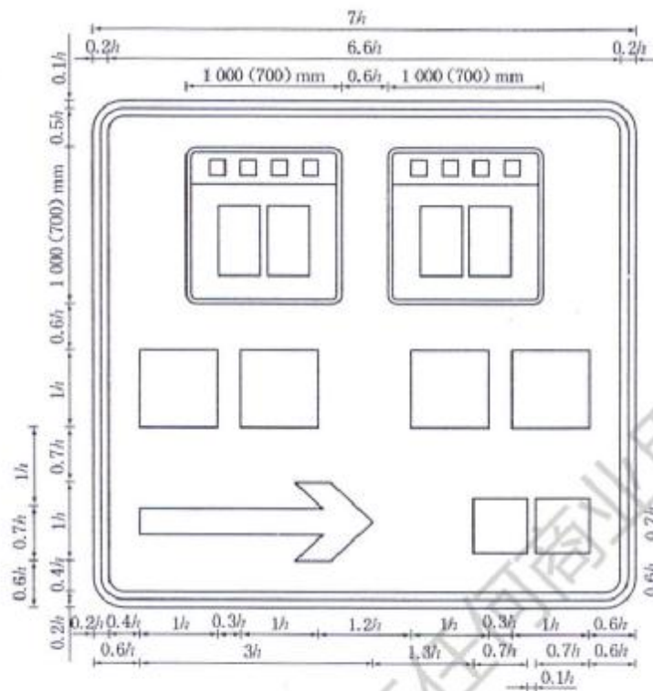
图 D.46 [图 251d)、e)]
