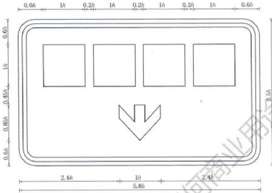
图 D. 118 [图 294c]
