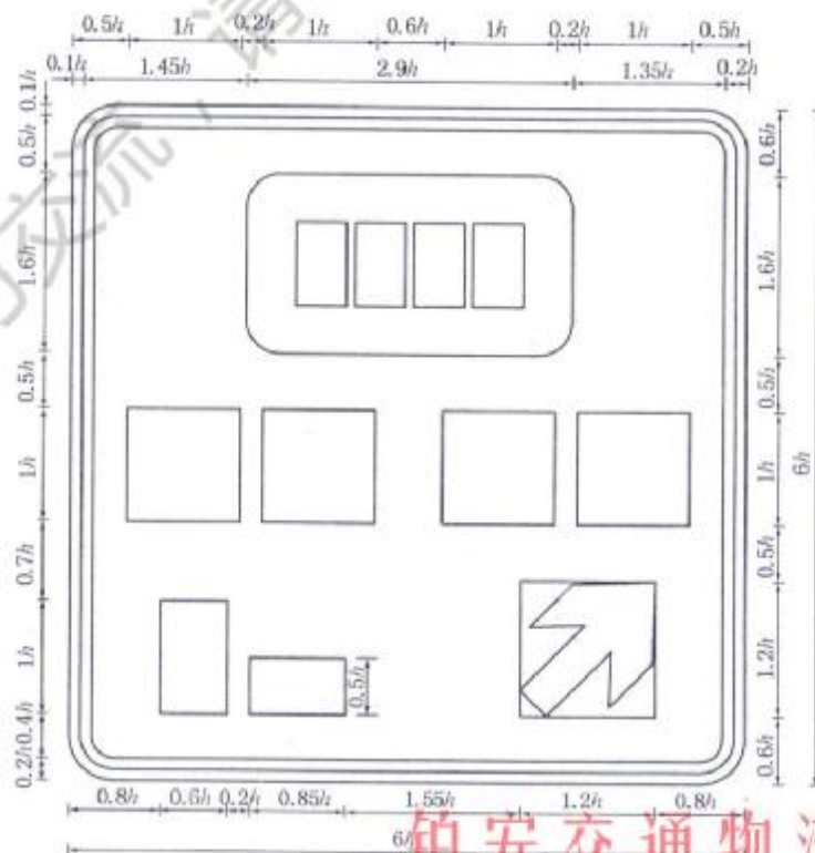
图 D.62 [图 261a)、b)]
