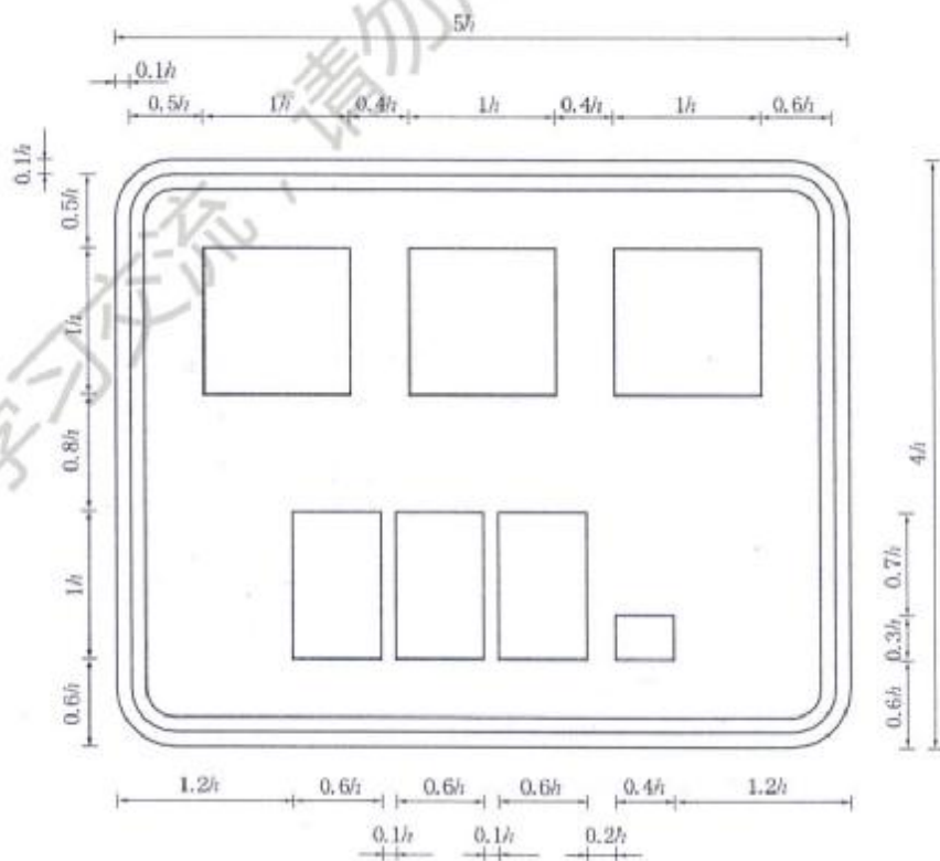
图 D.97 [图 283c)]
