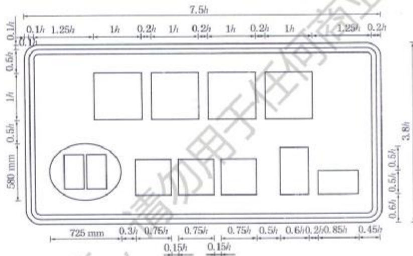
图 D.58 [图 259c)]
