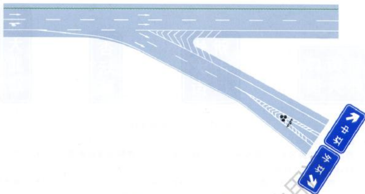
图 200 分岔处标志设置例
