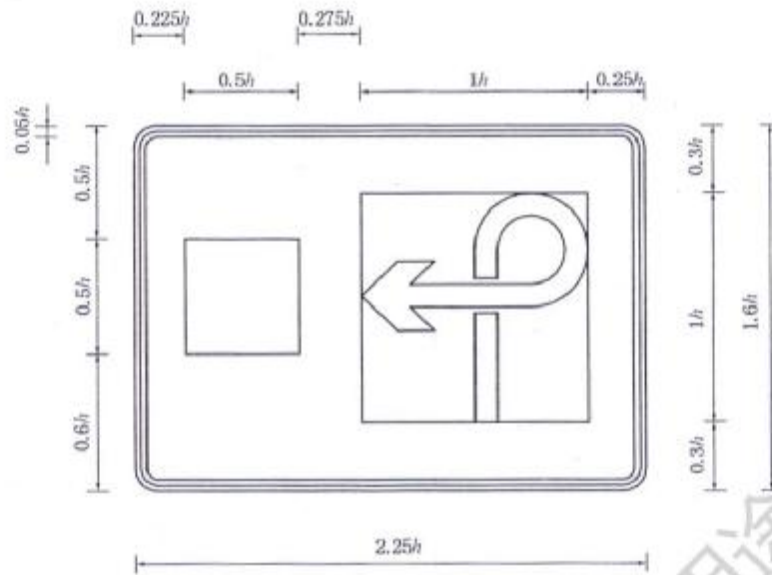
图 D.124 [图 297c]
