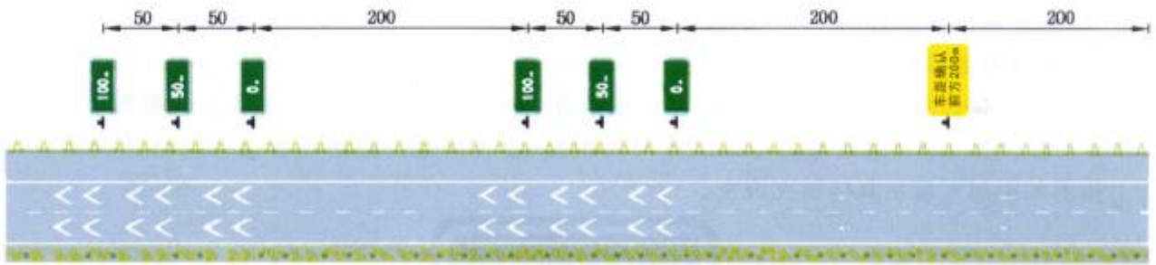
图 277 车距确认标志设置示例
